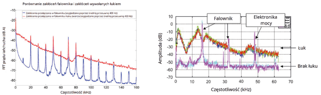
Rysunek 4: Przykłady widma częstotliwości z łukiem (czerwone krzywe) i bez (niebiesko-fioletowe krzywe) [7, 9].
