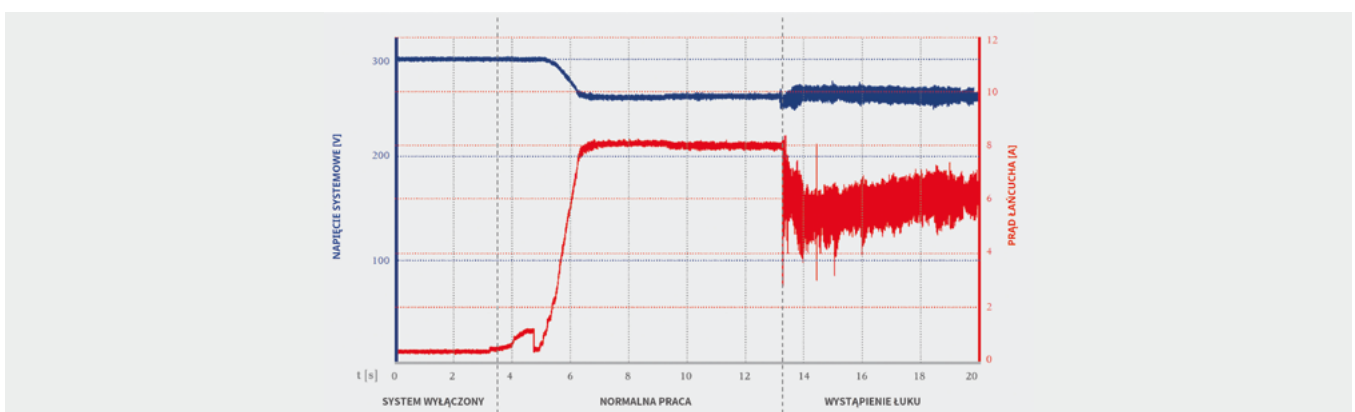
Rysunek 3: Sygnał napięcia i prądu w systemie fotowoltaicznym w dziedzinie czasu, przed i podczas łuku.
